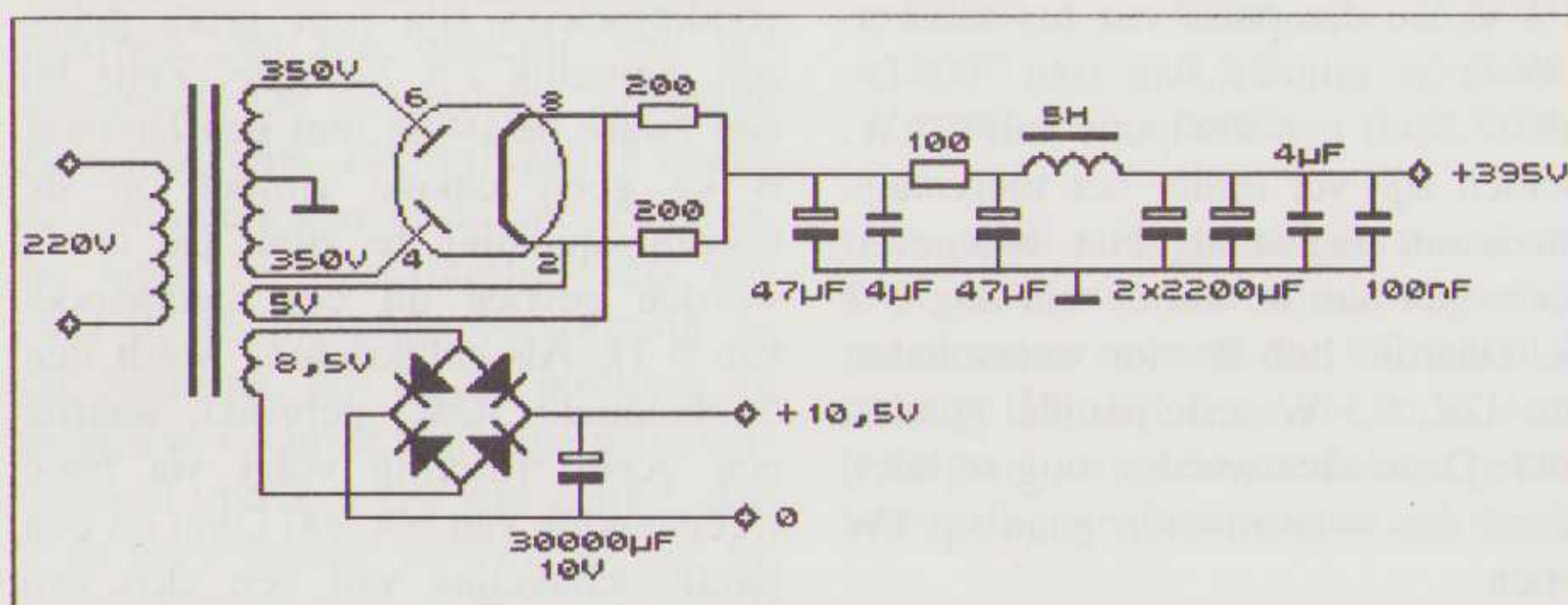
Fig. 1b. De voeding van de versterker
